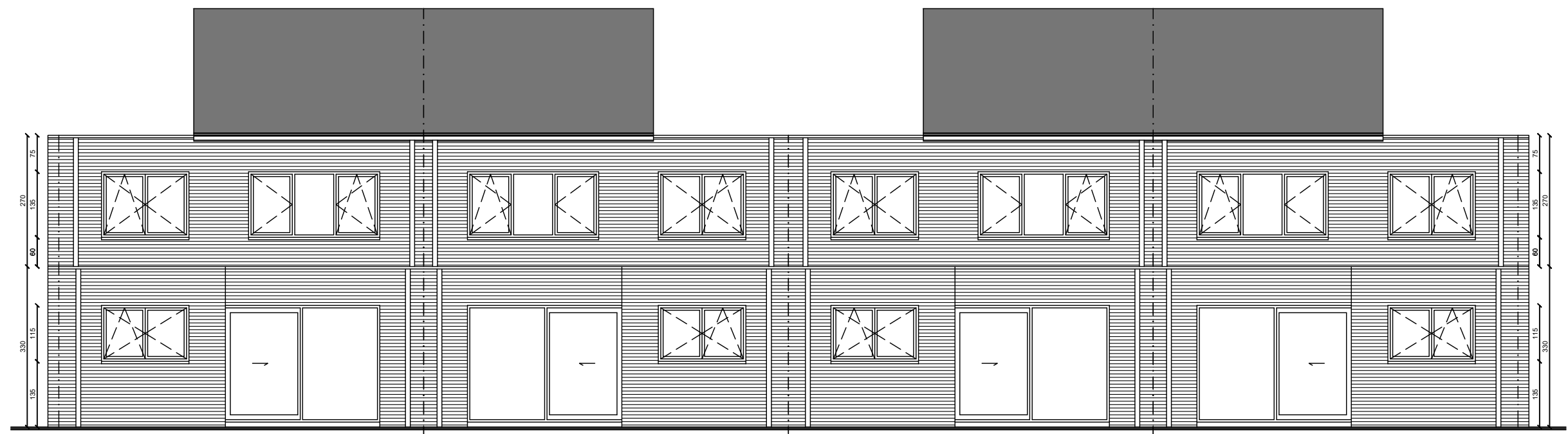
blok 3 achtergevel
