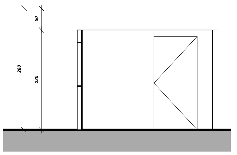
Voorgevel tuinhuis (principe) SCHAAL: 1:50
