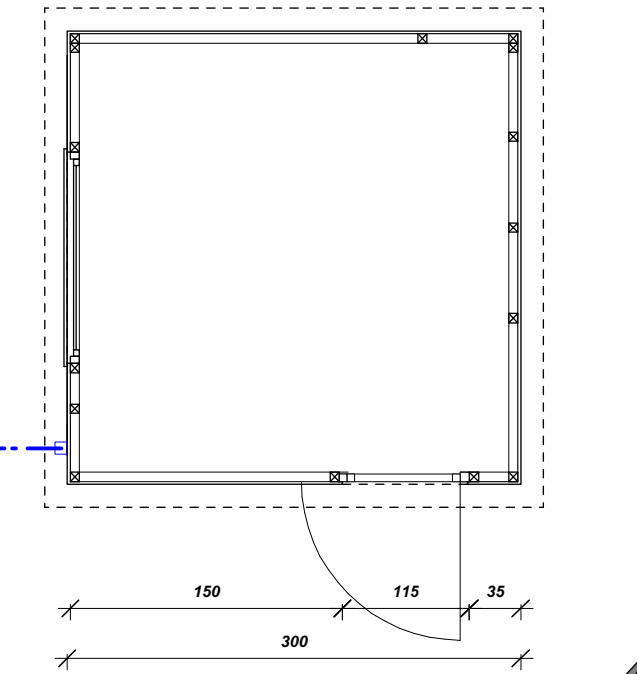
grondplan tuinhuis (principe) SCHAAL: 1:50
