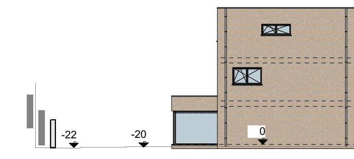
Terreinprofiel A SCHAAL: 1:250
