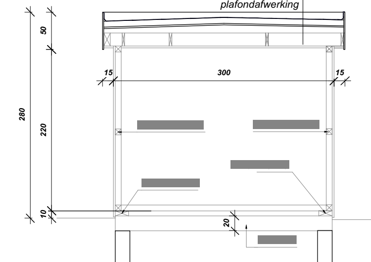
Doorsnede AA tuinhuis (principe) SCHAAL: 1:50
