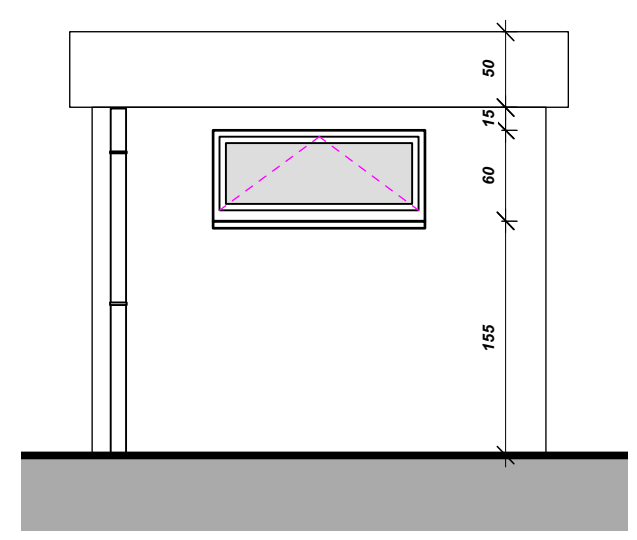
Zijgevel tuinhuis met raam (principe) SCHAAL: 1:50
